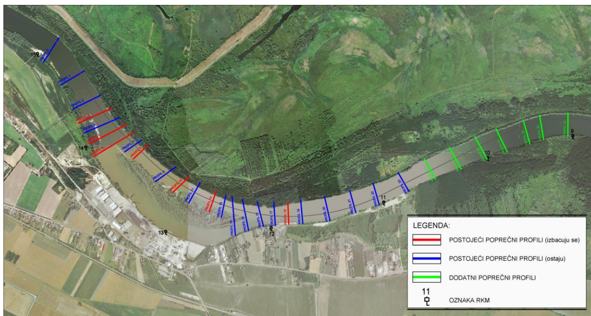
Slika.2: Pregledna situacija – položaj poprečnih profila
